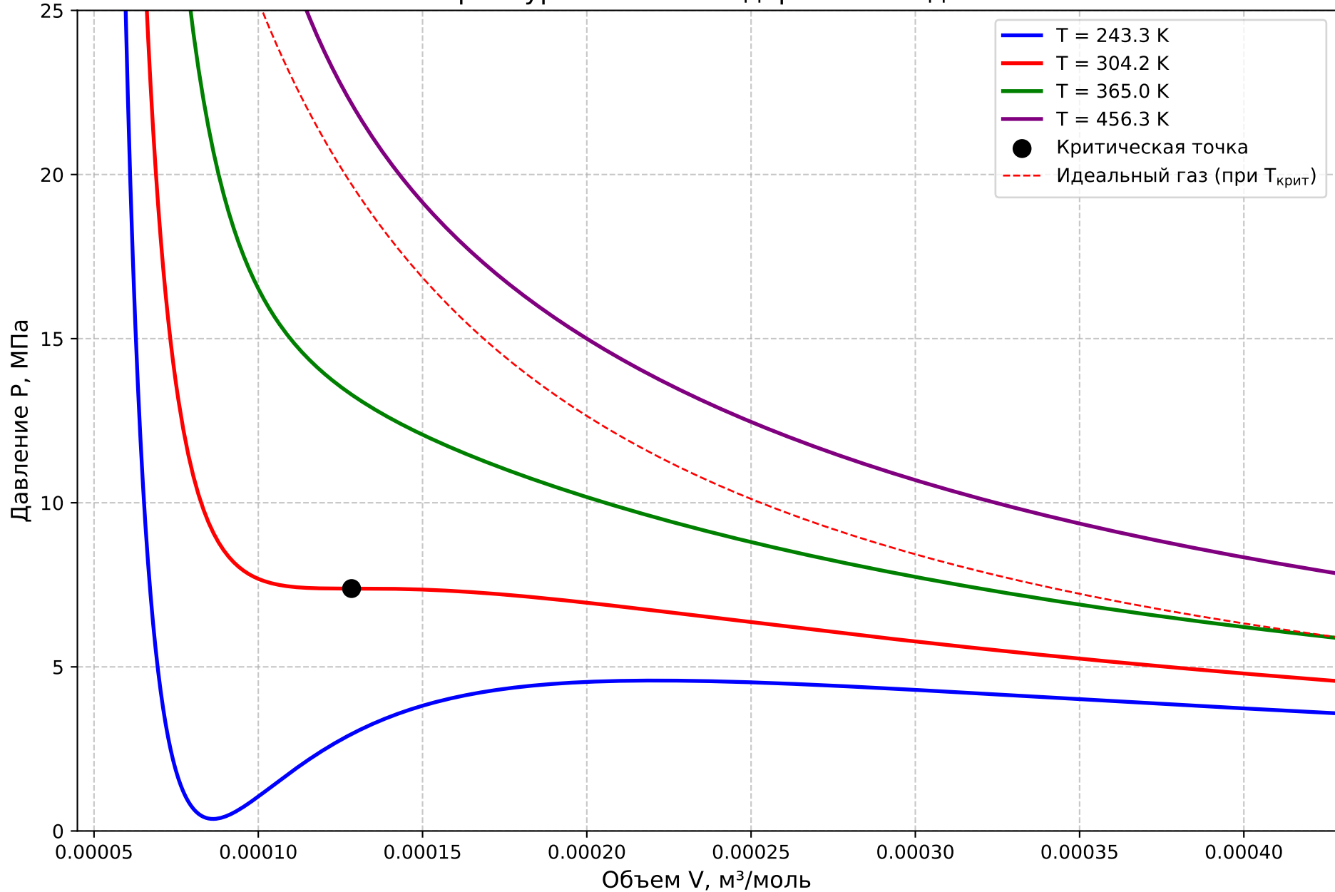
Изотермы уравнения Ван-дер-Ваальса для CO 2
